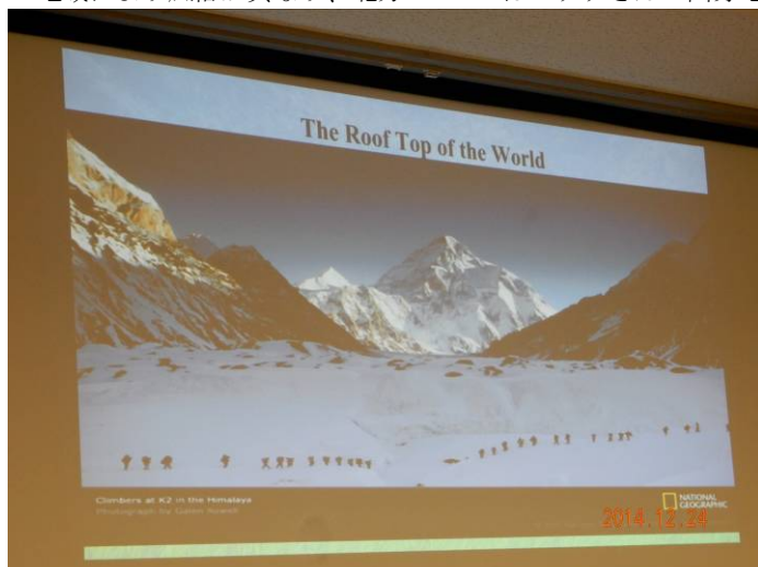
世界の屋根のカラコルム山脈。中央の山が K2
